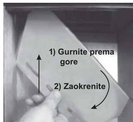
Slika. 17: Skinite zaštitni lim plamena
